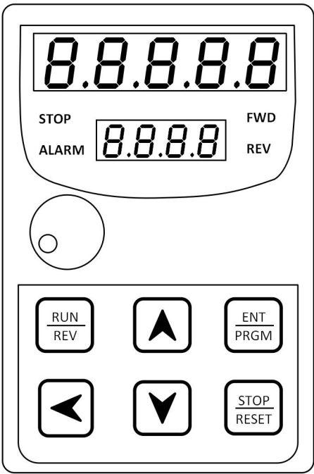
操作面板示意图（通用型）
