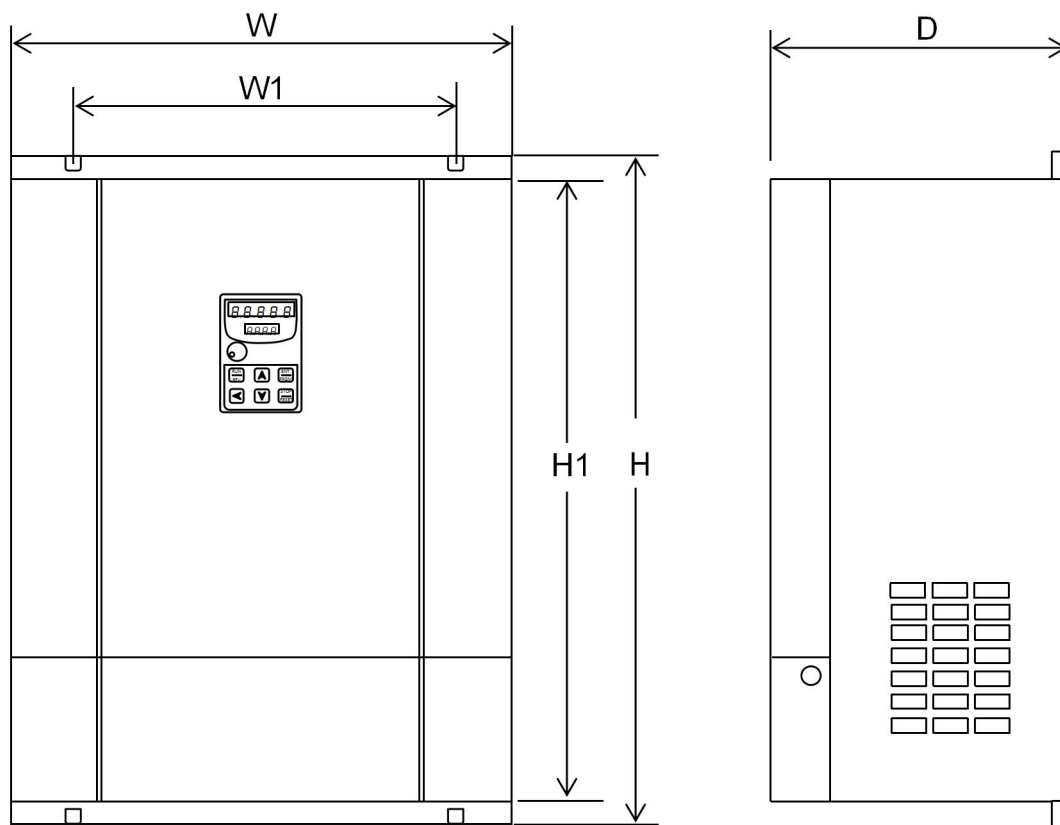
通用型外型图(45KW 以上)
