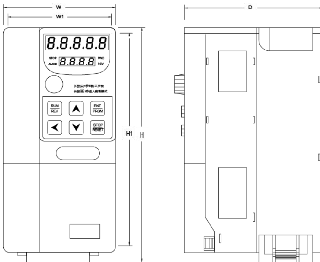
通用型外型图(5.5-37KW)
