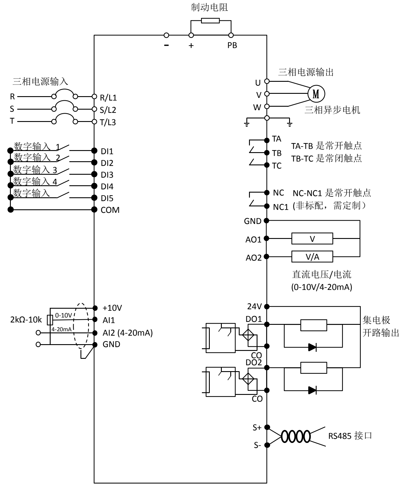
900 系列通用型三相 380V 端子接线图：
