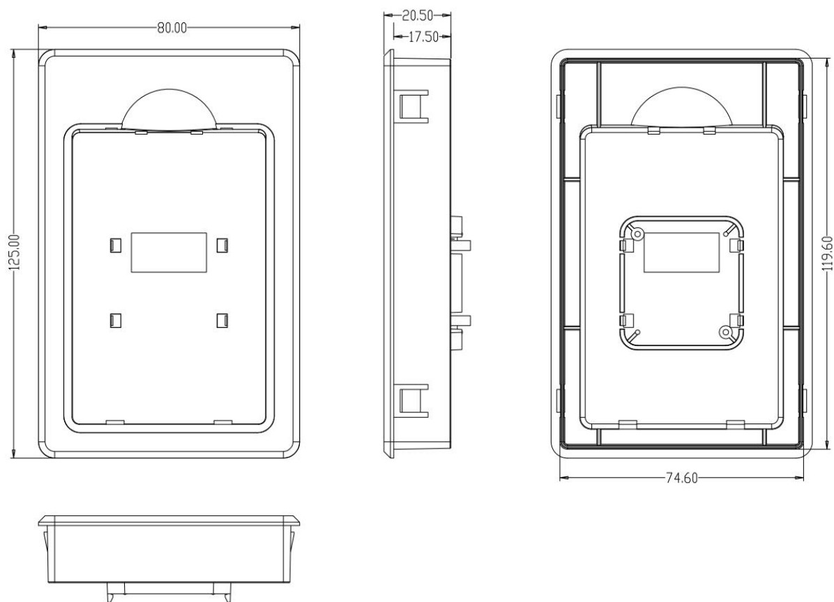
托盘外形尺寸图
